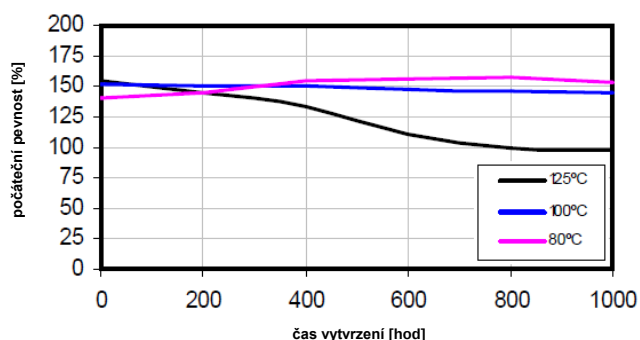
Rychlost vytvrzování
