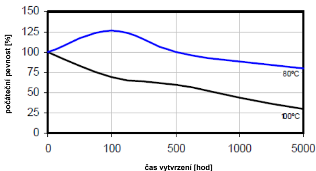
Rychlost vytvrzování
