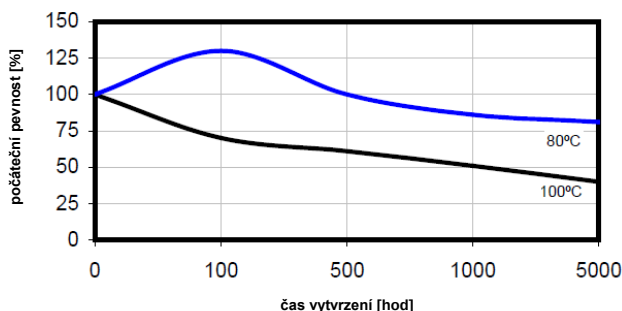
Rychlost vytvrzování
