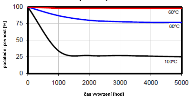
Rychlost vytvrzování
